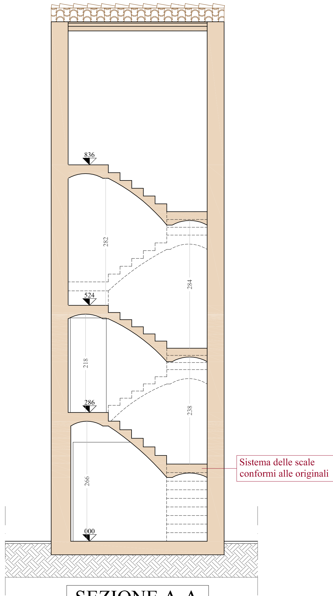
SEZIONE A-A
