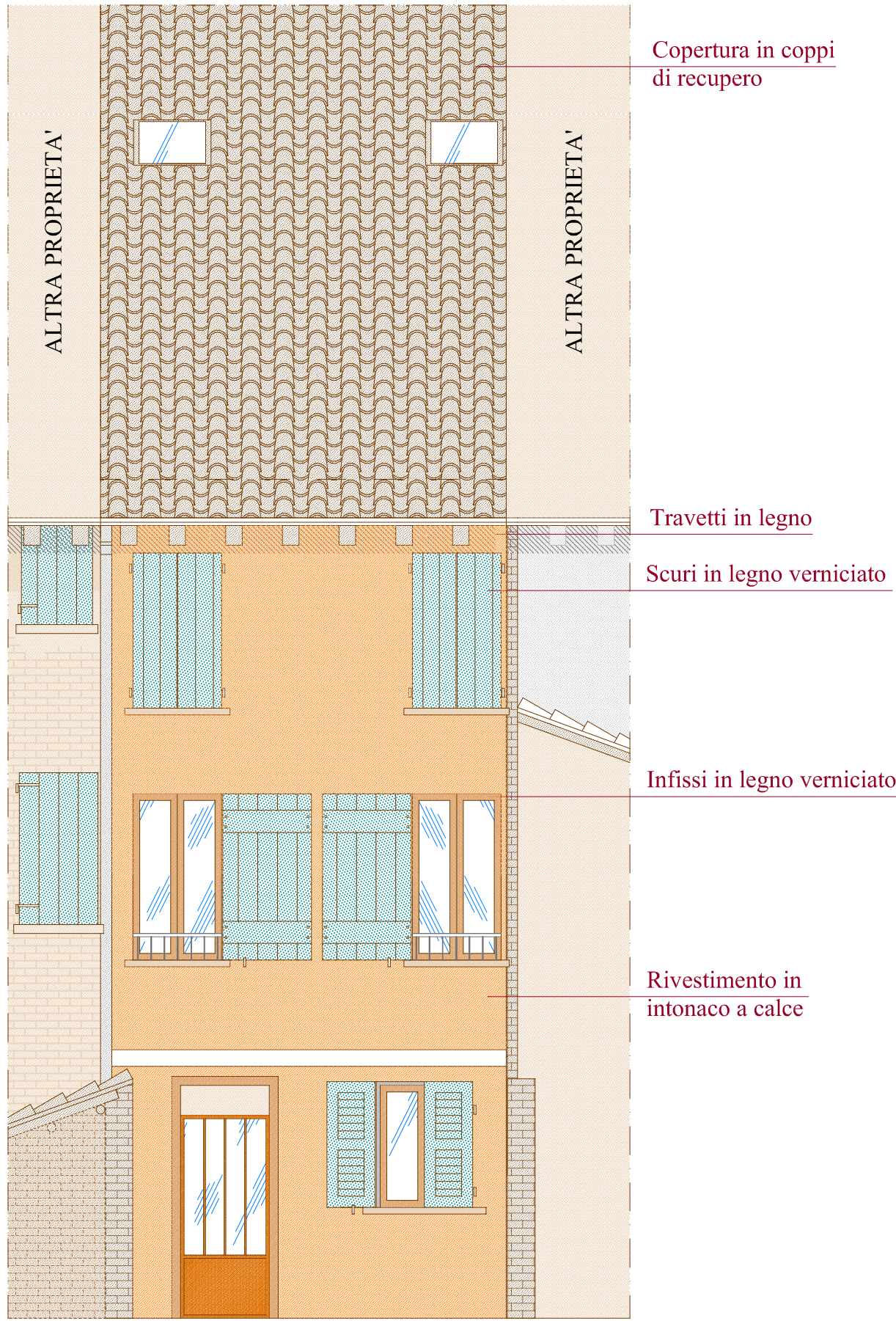
PROSPETTO RETRO
