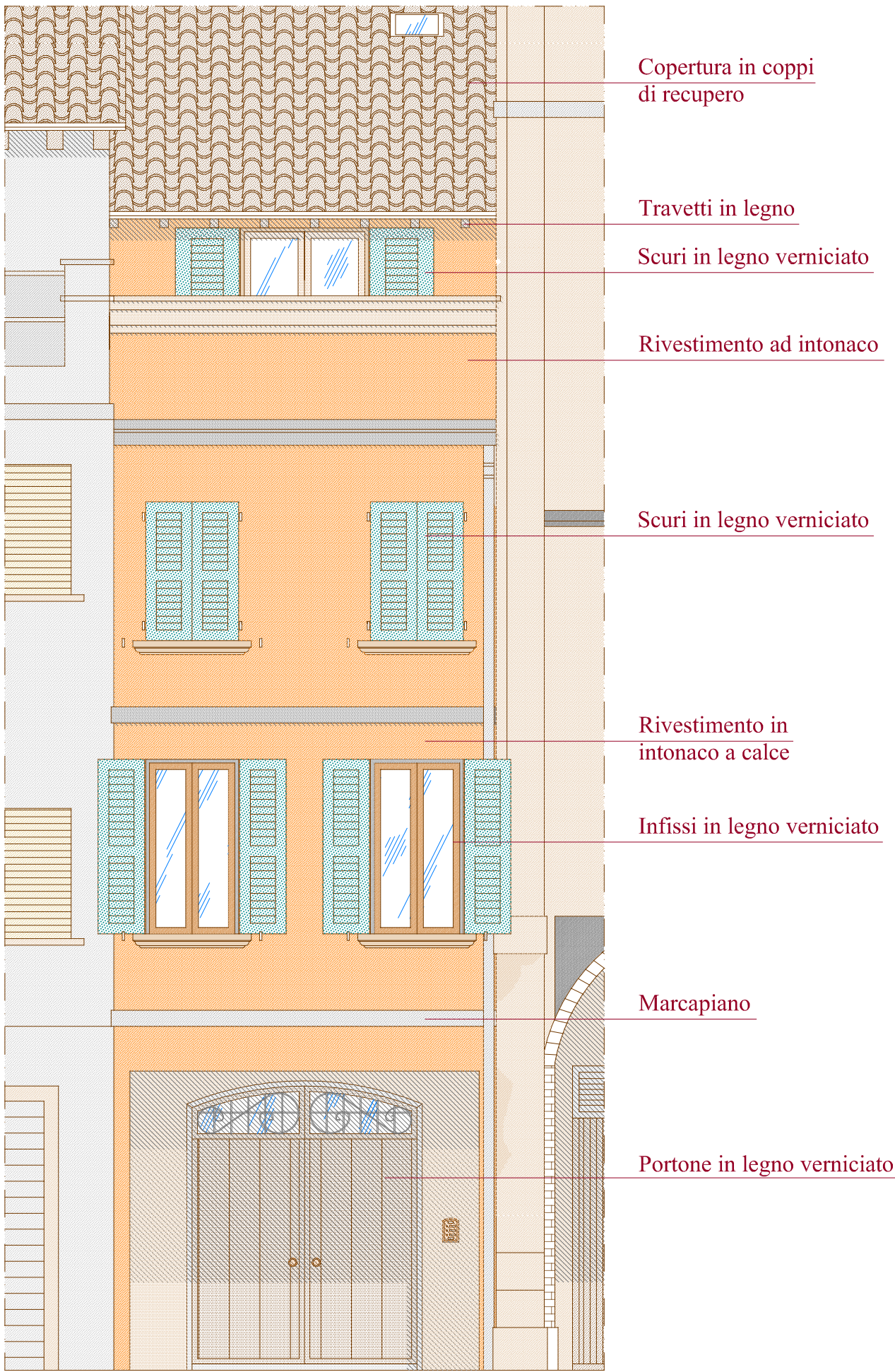
PROSPETTO FRONTE
